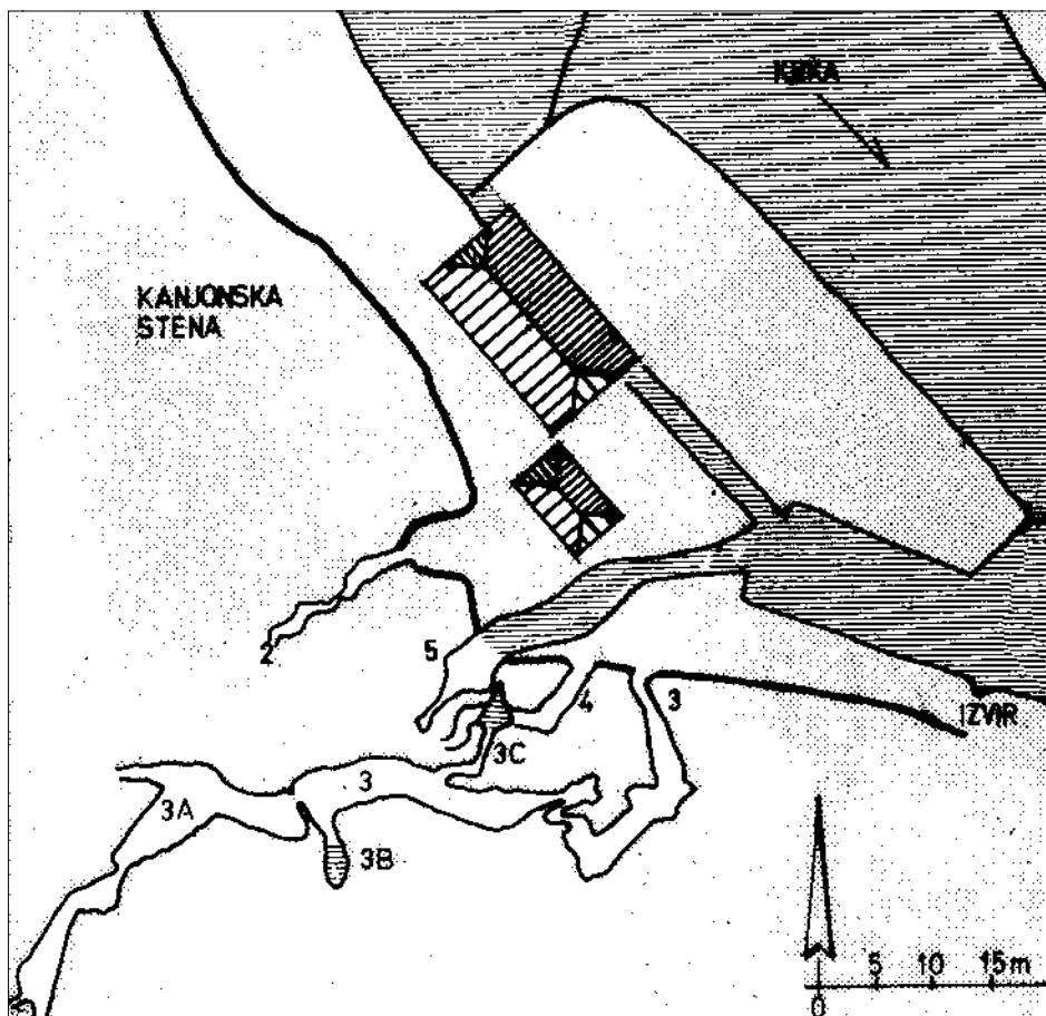
Jame ob izviru Šice: 2: Zgornja jama, 3: Črničkova jama (3A - Blatni rov, 3B - Vodnjak, 3C - Jezero), 4: Srednja jama, 5: Bruhalnik za Javornikovo žago.
